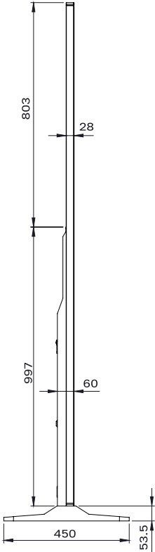
СХЕМА ДИСПЛЕЯ (ВИД СЛЕВА)
